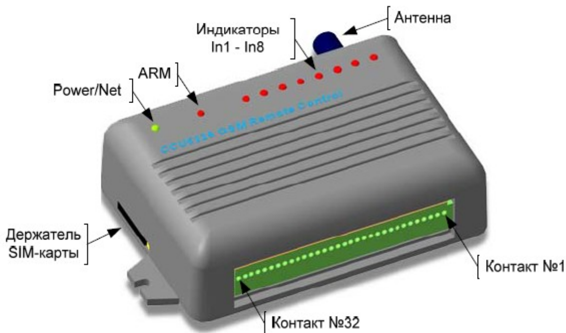
Рисунок 1. CCU6225 – основные элементы
