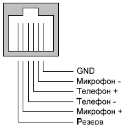
Рисунок 12. Назначение контактов телефонного разъема
