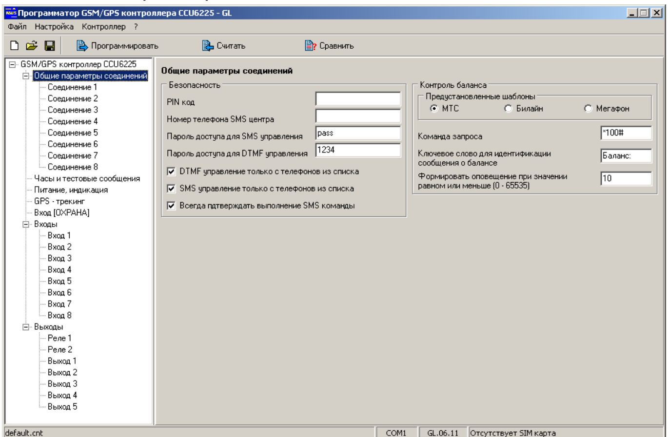
Рисунок 4. Общие параметры соединений
