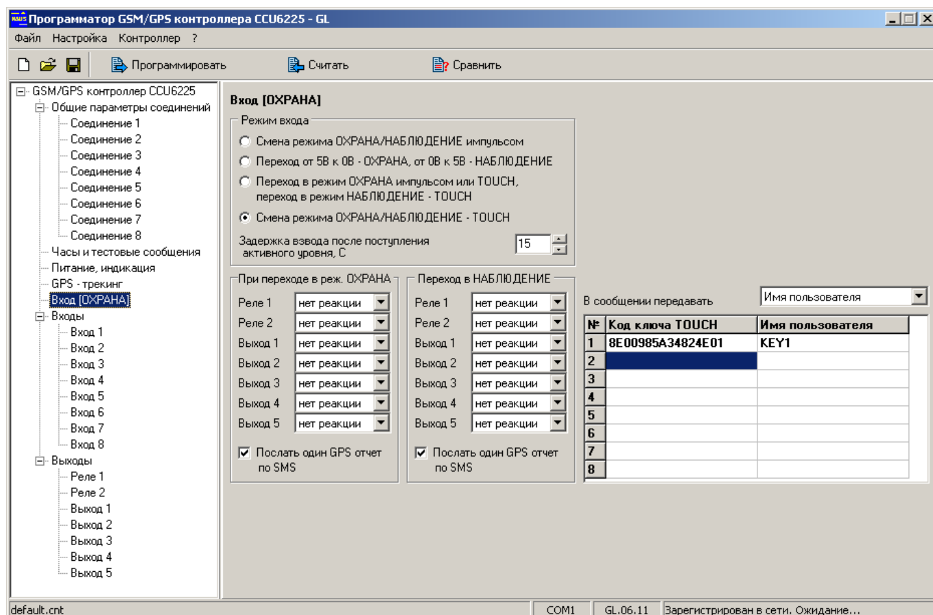
Рисунок 9. Настройка параметров входа "ОХРАНА"
