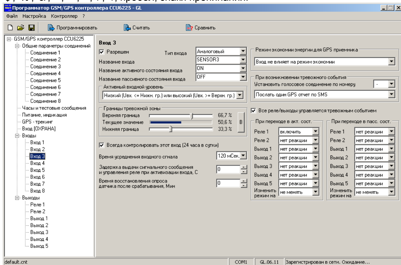
Рисунок 10. Типовая настройка параметров входа
