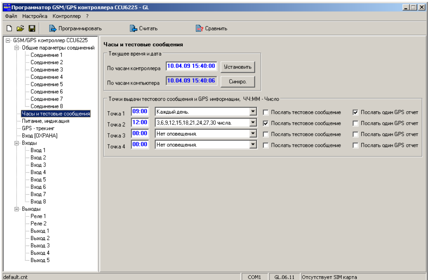
Рисунок 6. Часы и тестовые сообщения
