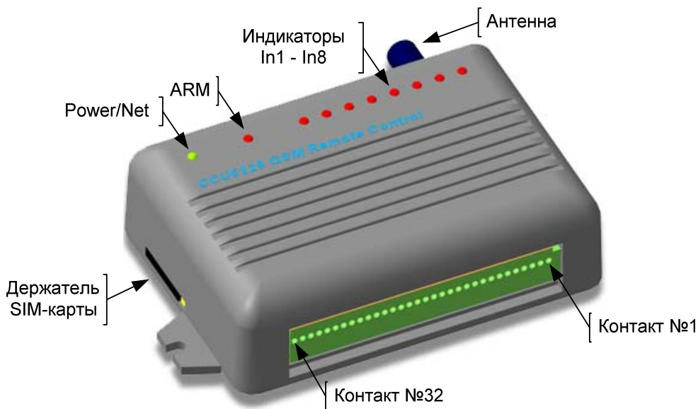
Рисунок 2. CCU6225 – основные элементы
