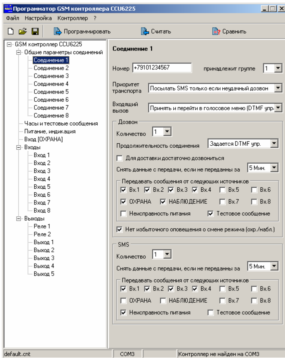
Рисунок 5. Параметры соединения
