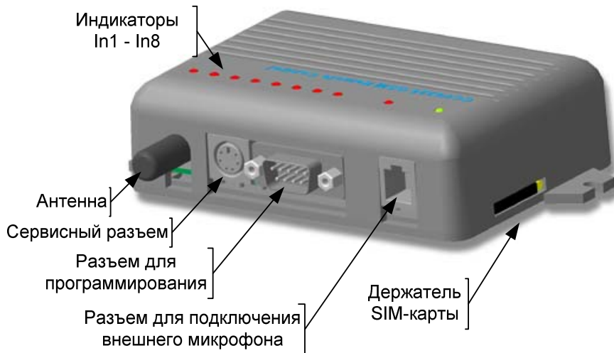
Рисунок 1. CCU6225 – основные элементы
