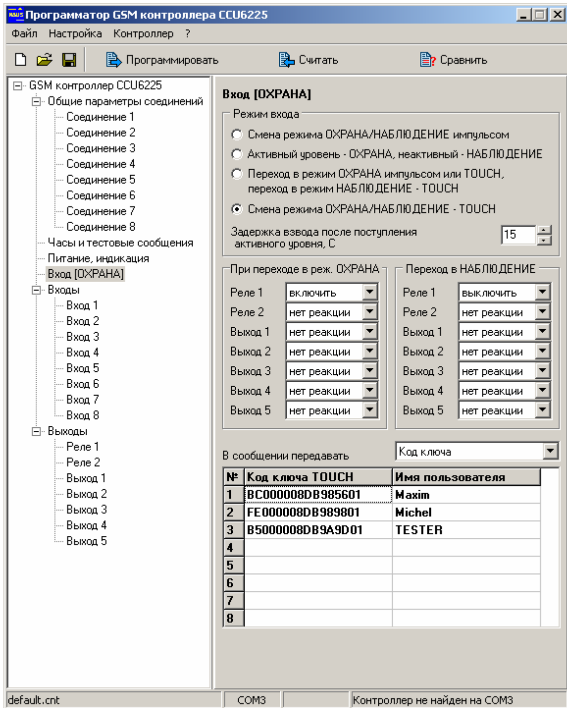
Рисунок 8. Настройка параметров входа "ОХРАНА"
