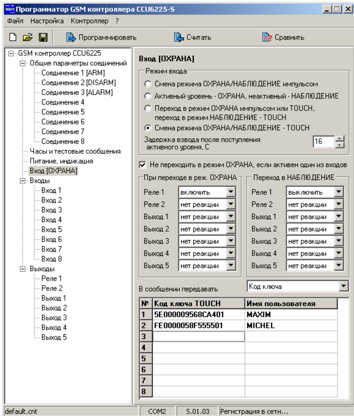
Рисунок 11. Настройка параметров входа "ОХРАНА"
