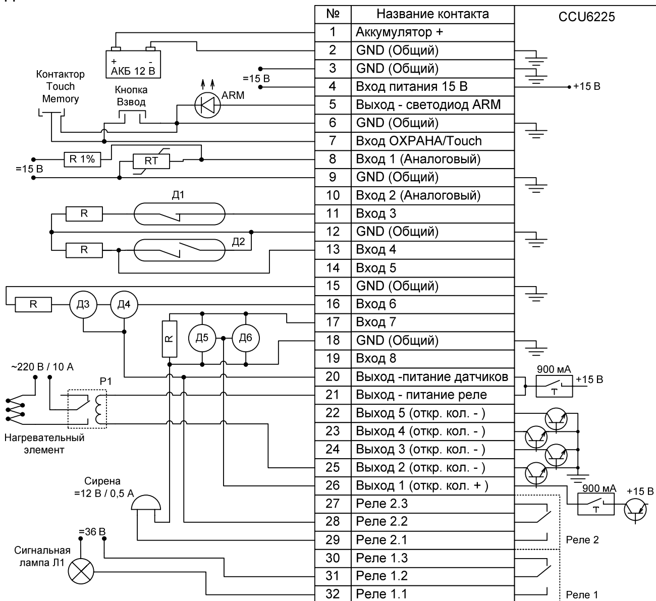
Рисунок 16. Схема подключения датчиков и других устройств
