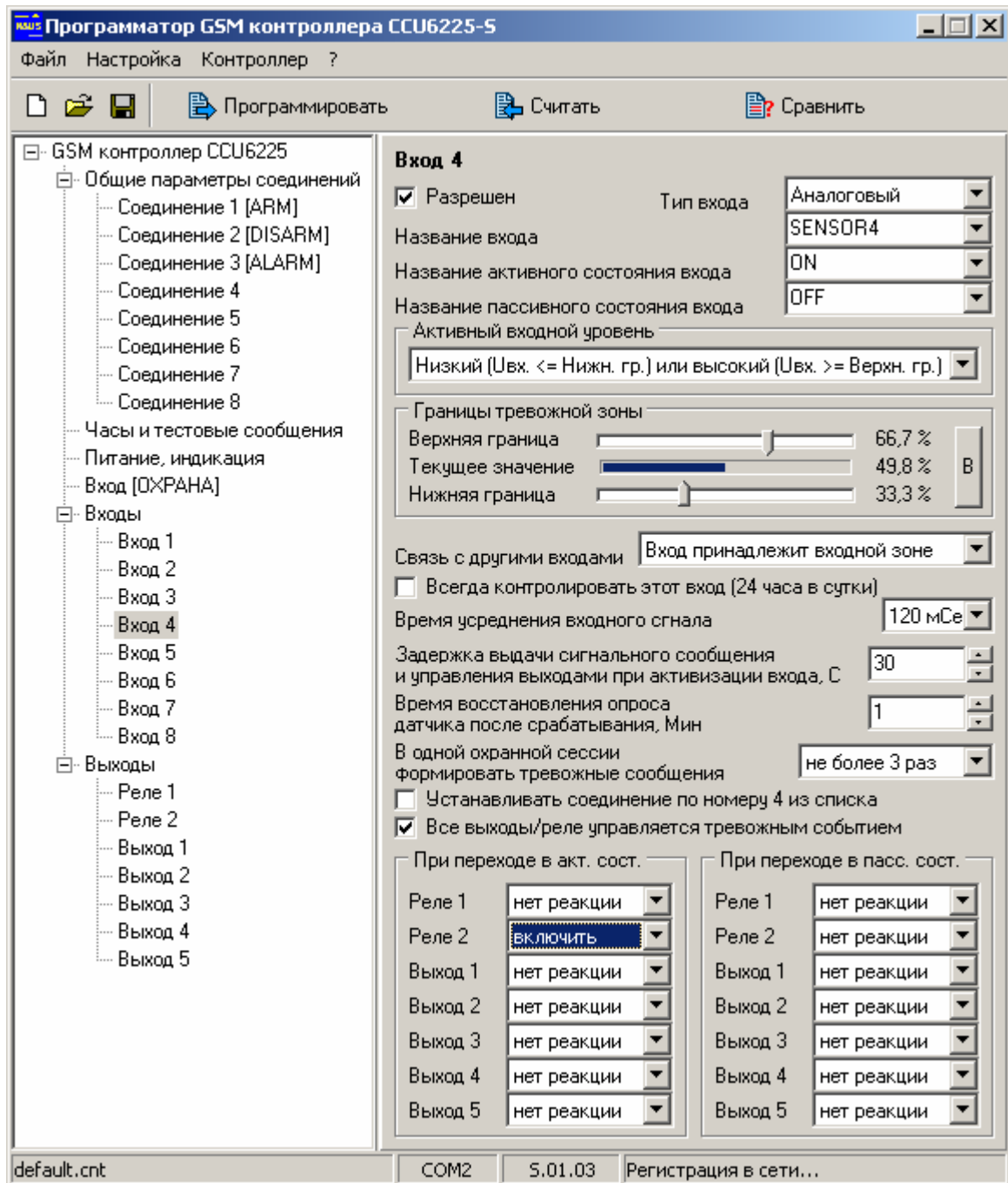
Рисунок 12. Типовая настройка параметров входа
