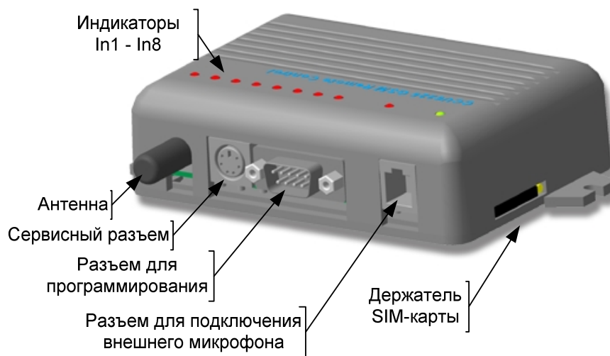
Рисунок 1. ССУ6225 – основные элементы
