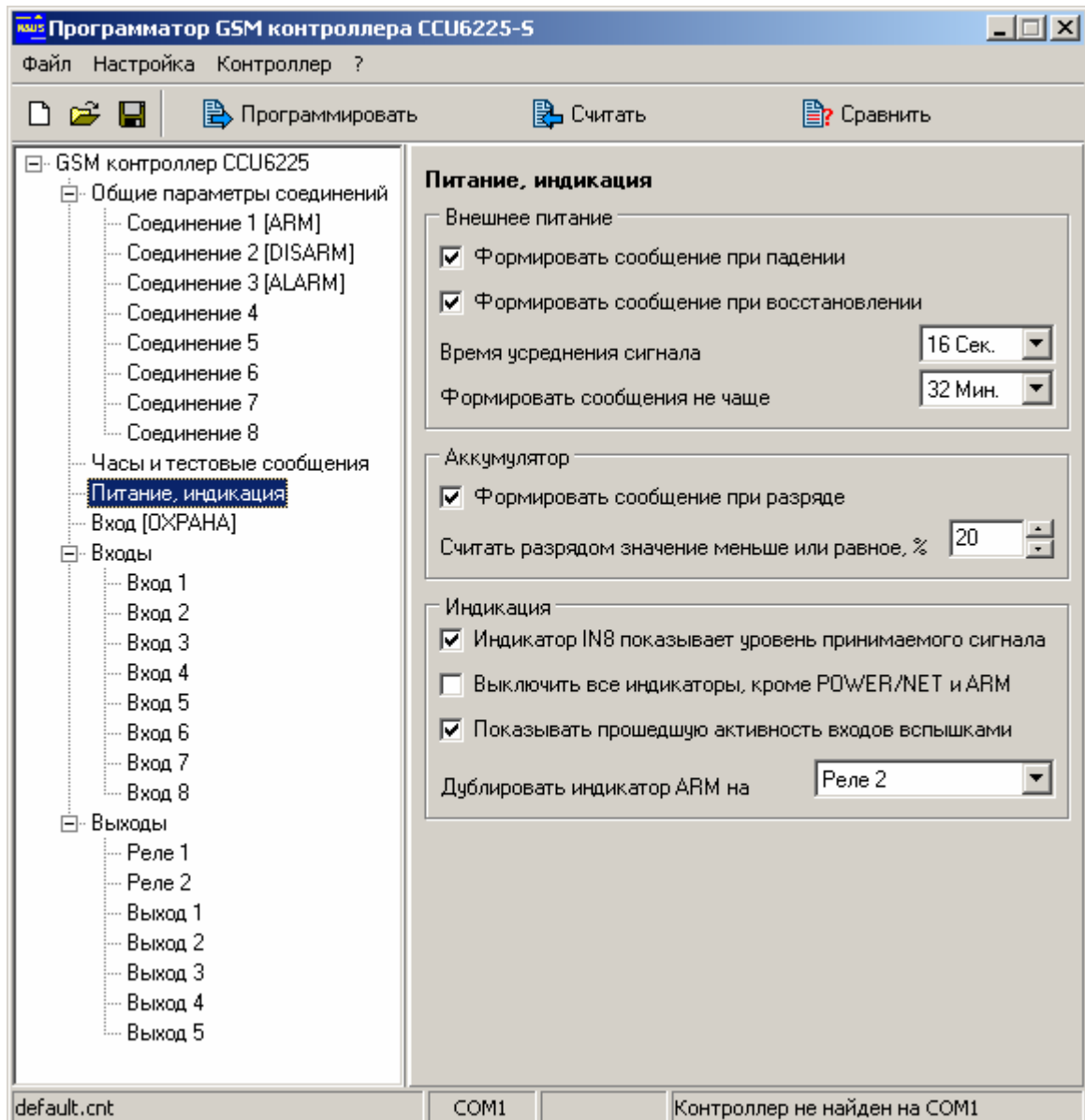
Рисунок 10. Сообщения формируемые при неисправности питания
