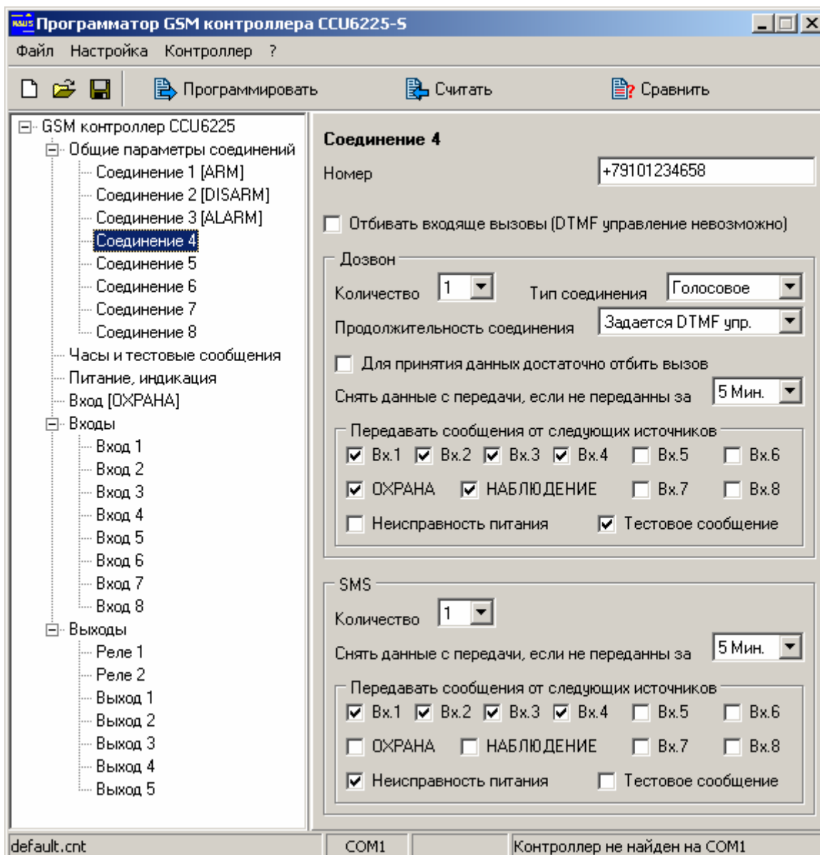
Рисунок 8. Параметры соединения общего назначения
