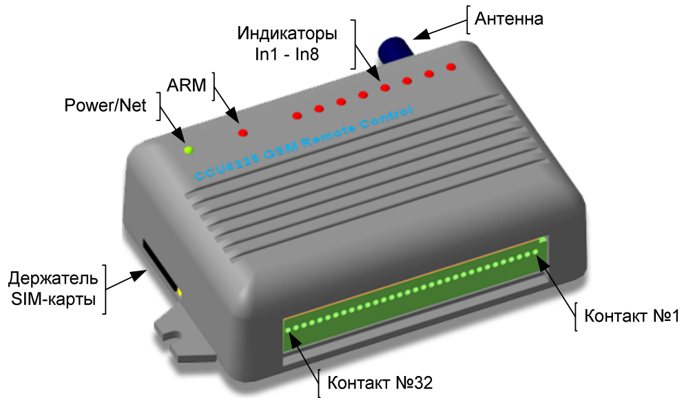
Рисунок 2. CCU6225 – основные элементы
