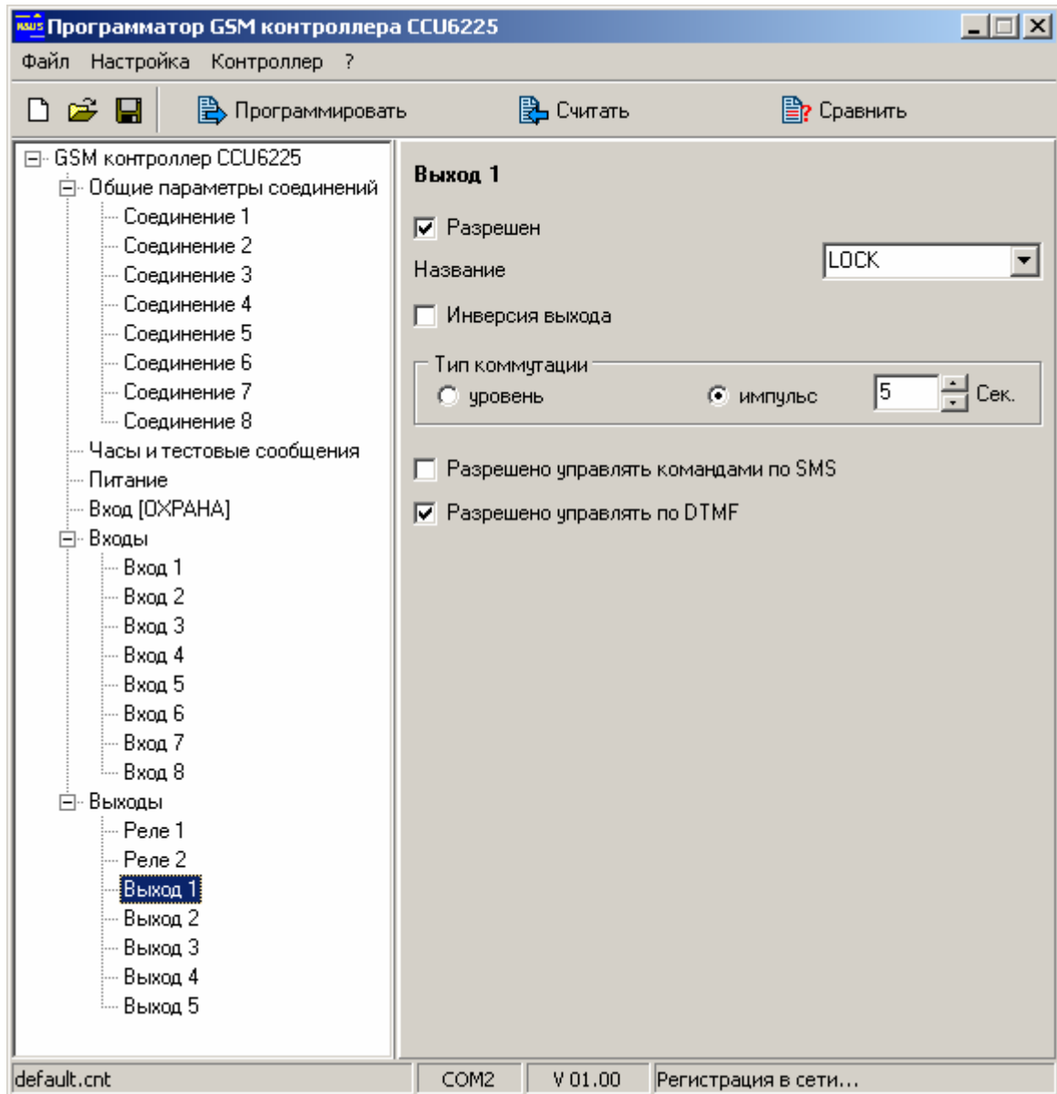
Рисунок 13. Типовая настройка параметров выходов
