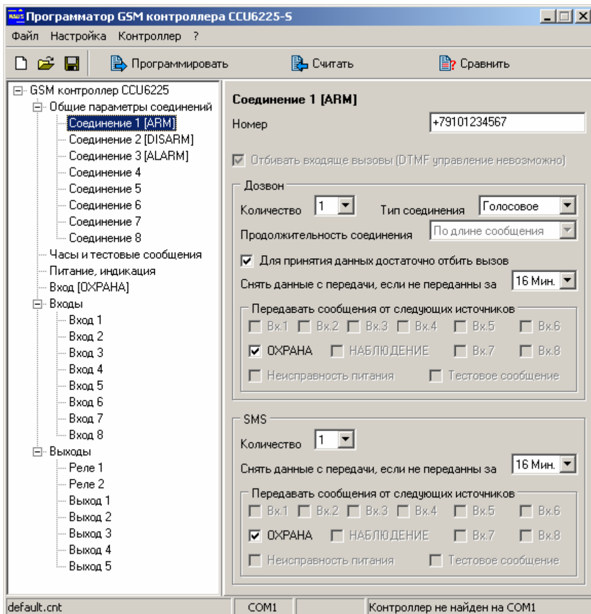
Рисунок 5. Параметры соединения "ARM"
